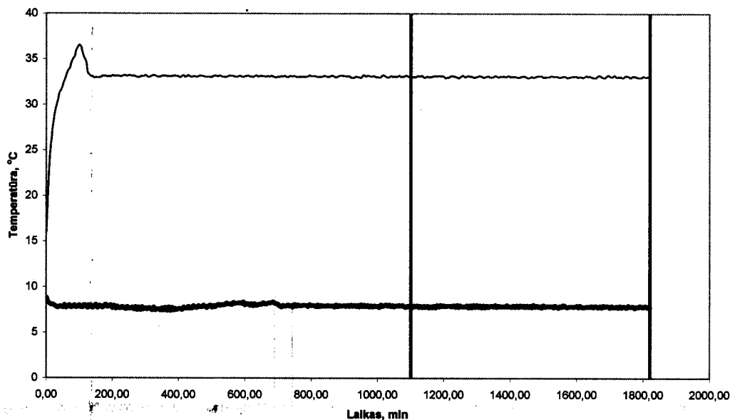
Temperatūrų grafikas
