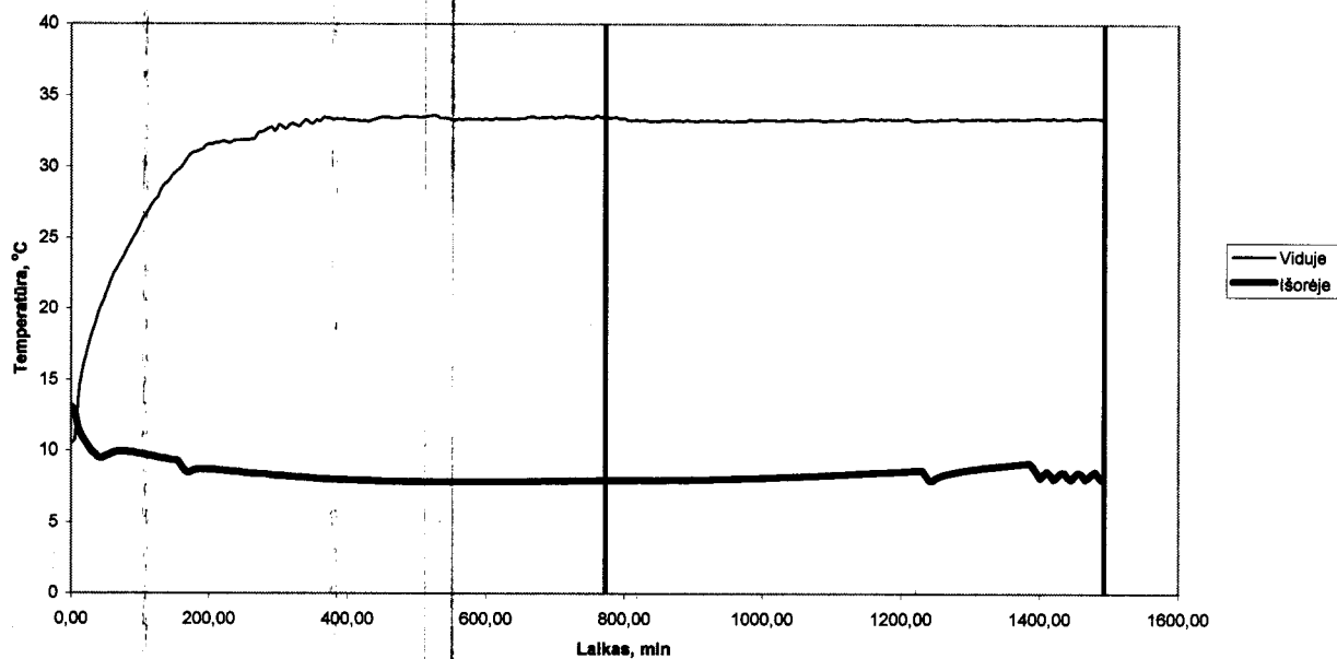
Temperatūrų grafikas
