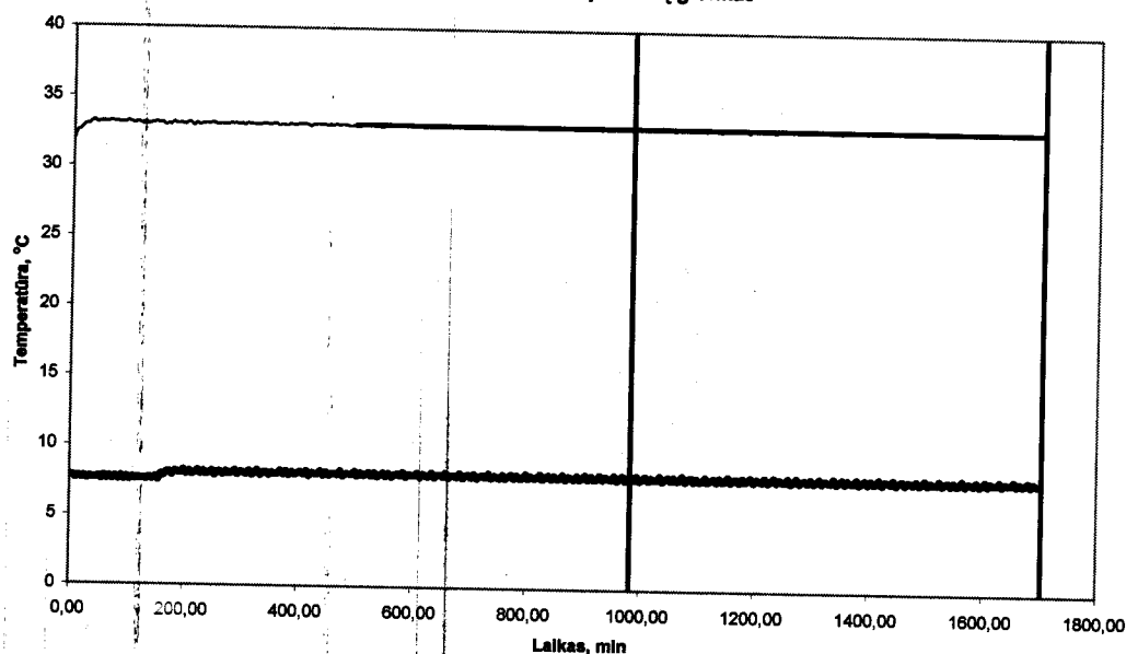
Temperatūrų grafikas
