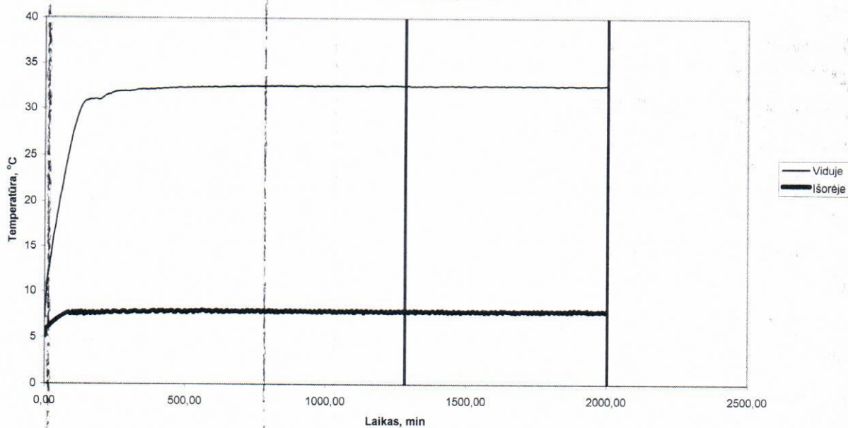
Temperatūrų grafikas
