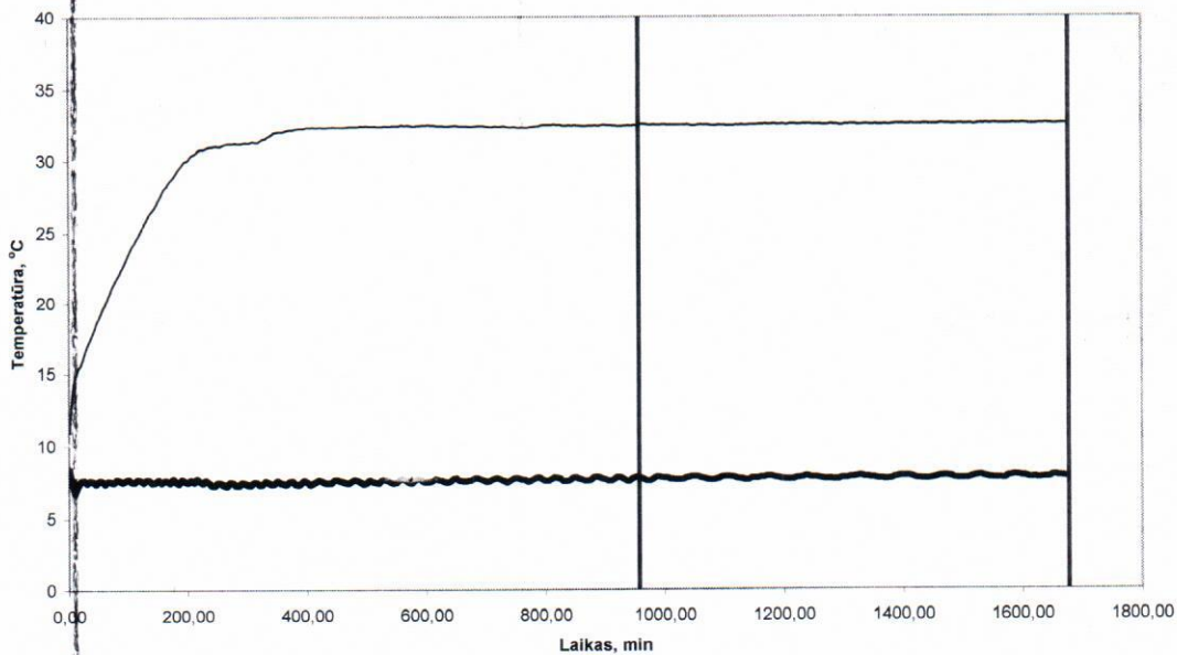
Temperatūrų grafikas
