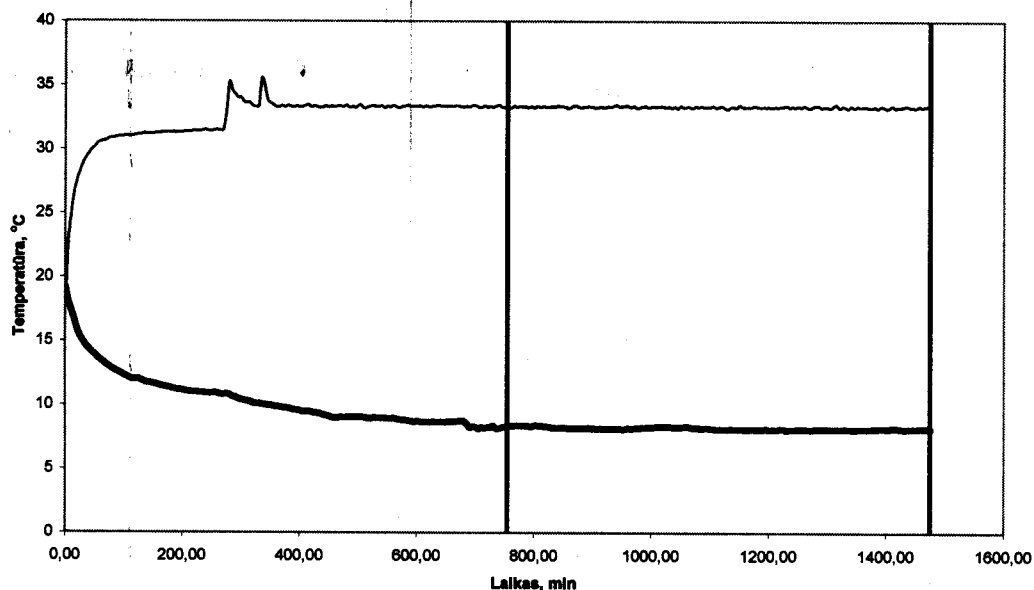
Temperatūrų grafikas
